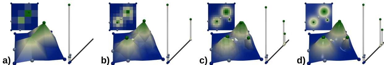
Fig. 1. Le sujet en une image – L’homologie persistante est un outil théorique puissant, qui permet en pratique d’introduire une mesure de bruit sur les structures topologiques, comme les singularités (sphères bleues et vertes) dans cet exemple de carte d’élévation. Cette mesure de bruit, appelée persistance , permet de visualiser et de mesurer des structures topologiques à plusieurs échelles d’importance et d’extraire efficacement et avec précision les structures d’intérêt dans un jeu de données. La persistance est souvent associée au diagramme de persistance (à droite sur ces exemples), qui donne une représentation visuelle de la distribution des structures topologiques (ici des singularités) en fonction de leur plage de valeur dans les données. Ces diagrammes, grâce à leur stabilité [10], jouent un rôle central en analyse topologique de données. Bien qu’il existe des algorithmes parallèles efficaces pour leur calcul [1, 18], ces approches demeurent couteuses en temps et dans de nombreuses applications, il peut être désirable d’obtenir uniquement une approximation du diagramme exact, mais en temps contrôlé. Dans ce stage, nous souhaitons répondre à ce problème en concevant une approche progressive ( coarse-to-fine ) pour le calcul de diagrammes de persistance, qui puisse fournir rapidement une approximation grossière mais fidèle du diagramme (a), pour ensuite la raffiner progressivement (b, c) vers le résultat exact (d).
