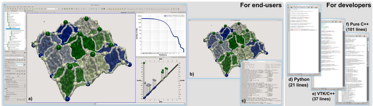
Fig. 1. TTK (the “Topology ToolKit” [38]) est une bibliothèque open-source écrite en C++ pour l’analyse topologique de données. Elle fournit plusieurs interfaces (C++ pure (f), VTK/C++ (e), Python (d)) pour répondre aux besoins de développeurs aux profils plus ou moins avancés. Pour les utilisateurs finaux, elle propose aussi des plugins pour la plateforme de visualisation open-source ParaView [44] (a) développée par l’entreprise Kitware [43]. TTK est disponible publiquement sous licence BSD depuis Avril 2017. Depuis, 11 institutions différentes ont contribué à son code (8 institutions académiques, 3 entreprises) et plus de 10,000 visiteurs uniques ont consulté son site web. Dans le cadre d’un projet européen (H2020-FET), nous recrutons un ingénieur de recherche en CDD pour une durée minimum d’un an, pour contribuer au maintien de TTK et au développement de nouvelles fonctionnalités.
